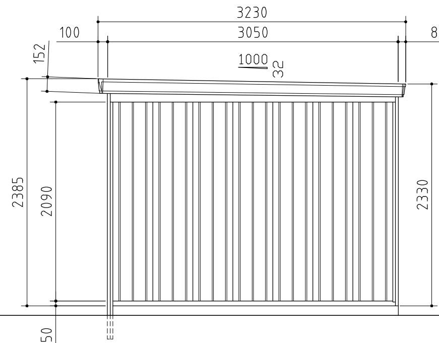
側面図
