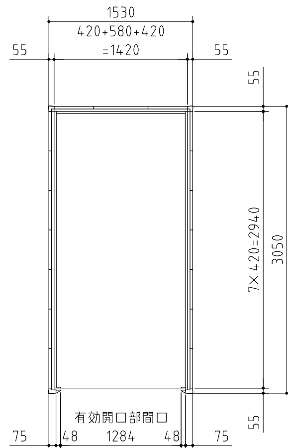
平面図
